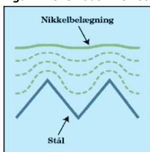
Figur 1 - Skematisk fremstilling af en nikkelbelægnings nivelleringssevne
